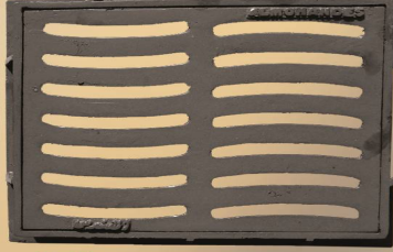
1 - 11 Grating and Frame size : 45 × 50 cm load : 1.5 tons to 90 tons أحمال من ١.٥ طن إلى ٩٠ طن غطاء صرف أمطار مقاس ٥٠ × ٤٥ سم
