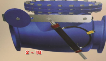
محابس عدم رجوع طراز سوينج هيدرولوكي وبدون Swing Type with & without Hydraulic Dampers
