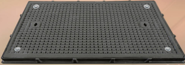
3 - 6 Square manhole cover Preventing Water Leakage Size: 40 x 40 - 50 x 50 - 60 x 60 - 70 x 70 80 x 80 - 90 x 90 - 100 x 100 cm load : 1.5 tons to 90 tons غطاء غرفة تفتيش مانع للمياه مقاس 70x70، 80x80، 90x90، 100x100 سم احمال 1,5 طن الى 90 طن
