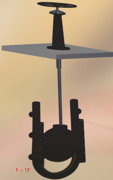
بوابة Rising Stem
